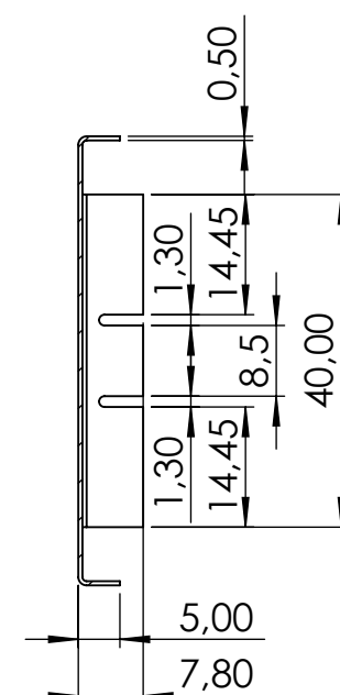
SEZIONE B-B
