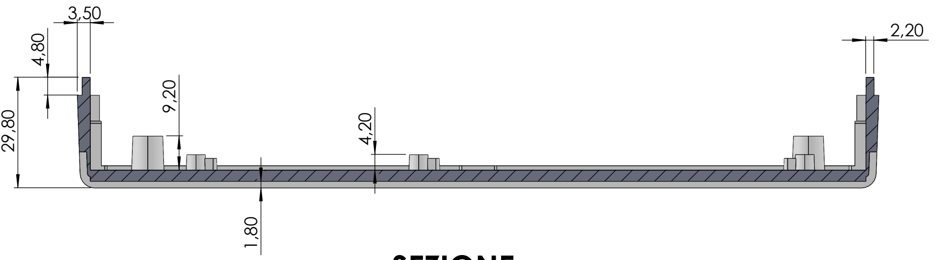
SEZIONE C-C
