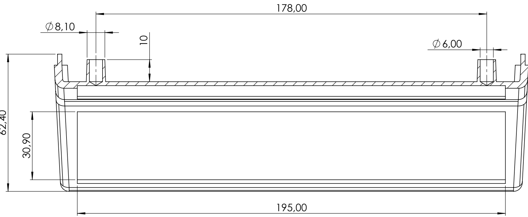
SEZIONE B-B
