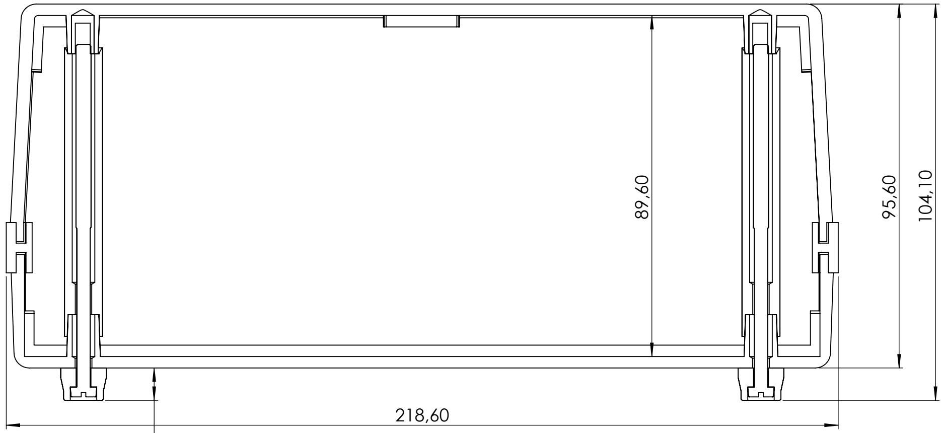
SEZIONE A-A
